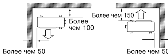
Вид сверху
