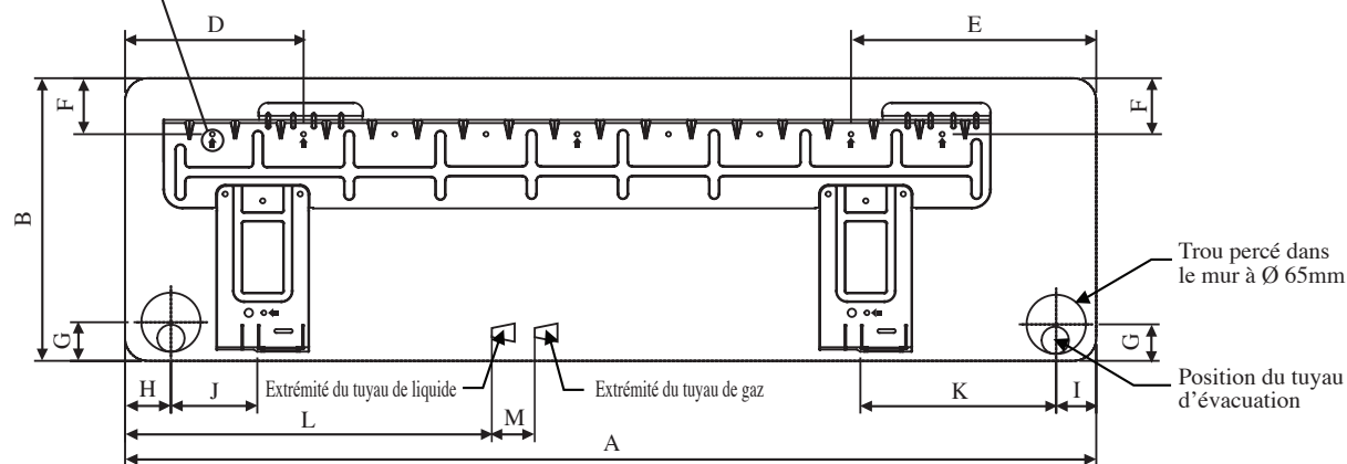
PLAQUE D'INSTALLATION FTYN50/60LV1B
