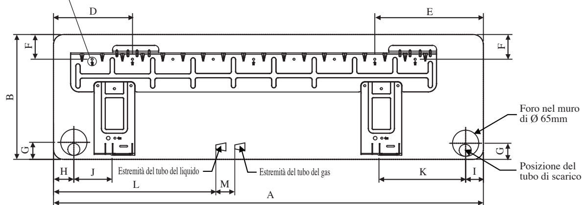
LASTRA DI INSTALLAZIONE FTYN50/60LV1B
