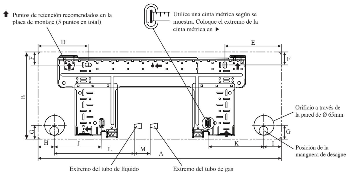
PLACA DE INSTALACIÓN FTYN25/35LV1B
