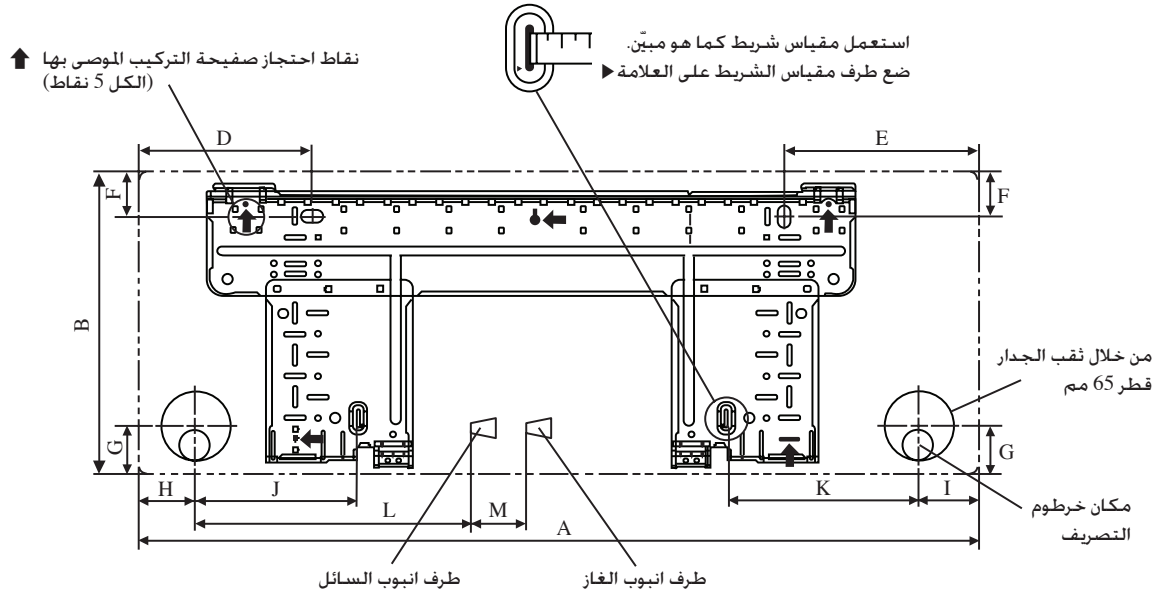
لوحة التركيب FTYN25/35LV1B
