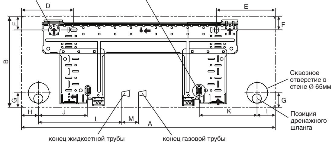
МОНТАЖНАЯ ПЛИТА FTYN25/35LV1B
