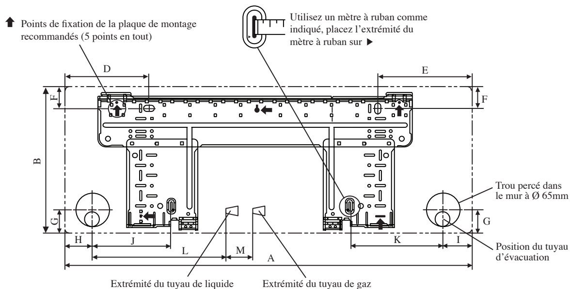
PLAQUE D'INSTALLATION FTYN25/35LV1B
