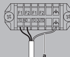
a Заземление
