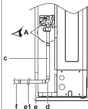
Вариант 3: подсоединение сбоку
