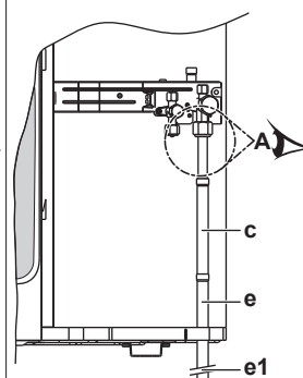
Вариант 4: подсоединение снизу
