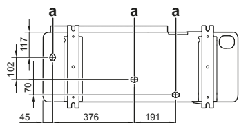
а Дренажные отверстия
